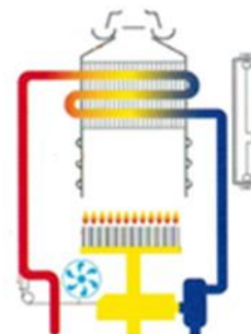
DIAGRAMA FUNCIONAL
