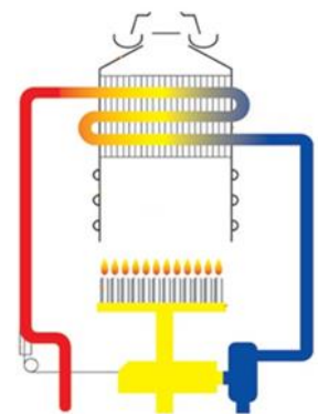
DIAGRAMA FUNCIONAL
